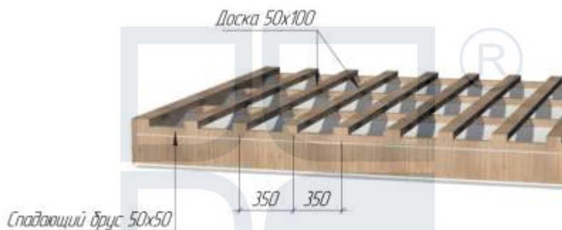
Рис.2 Схема обрешетки
