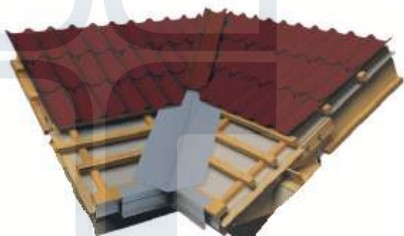
Рис.3 Крепление ендов
