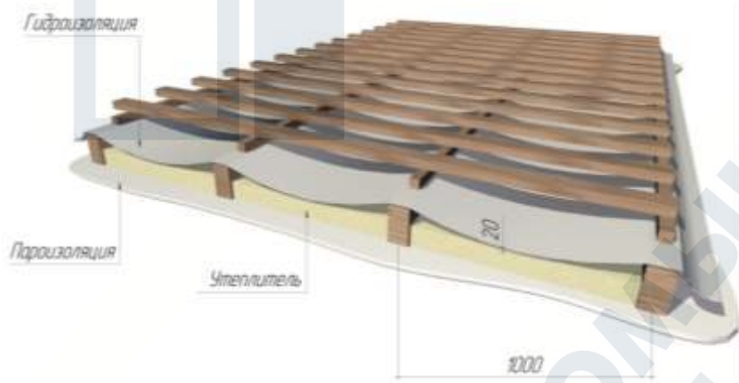
Рис.1 Состав теплой кровли
